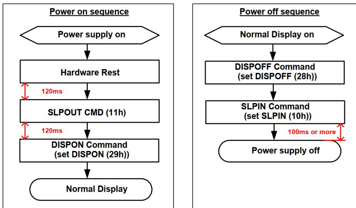
电源接通/断开顺序框图
